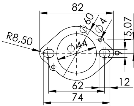
S.s. Flange Cod.204448R
